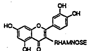
RUTIN
